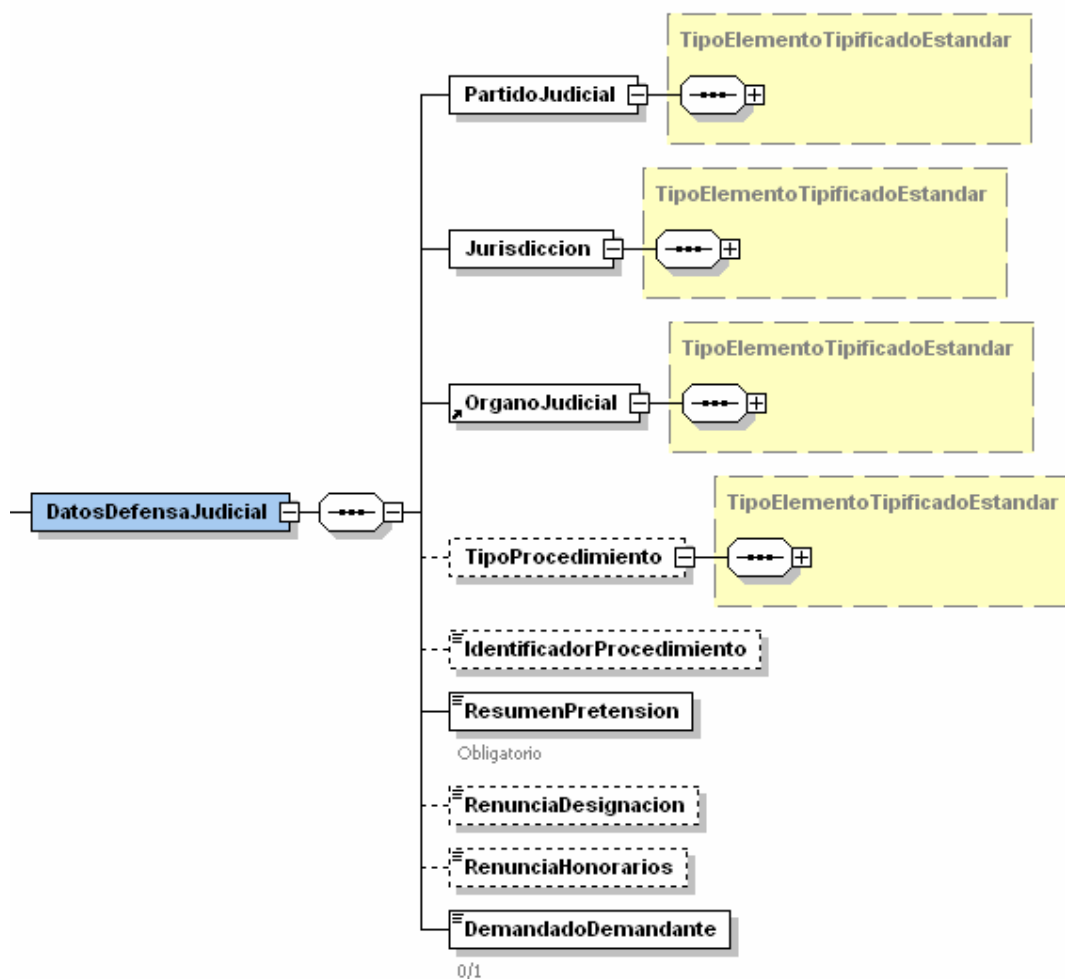
Figura 14. XSD-DatosDefensaJudicial
