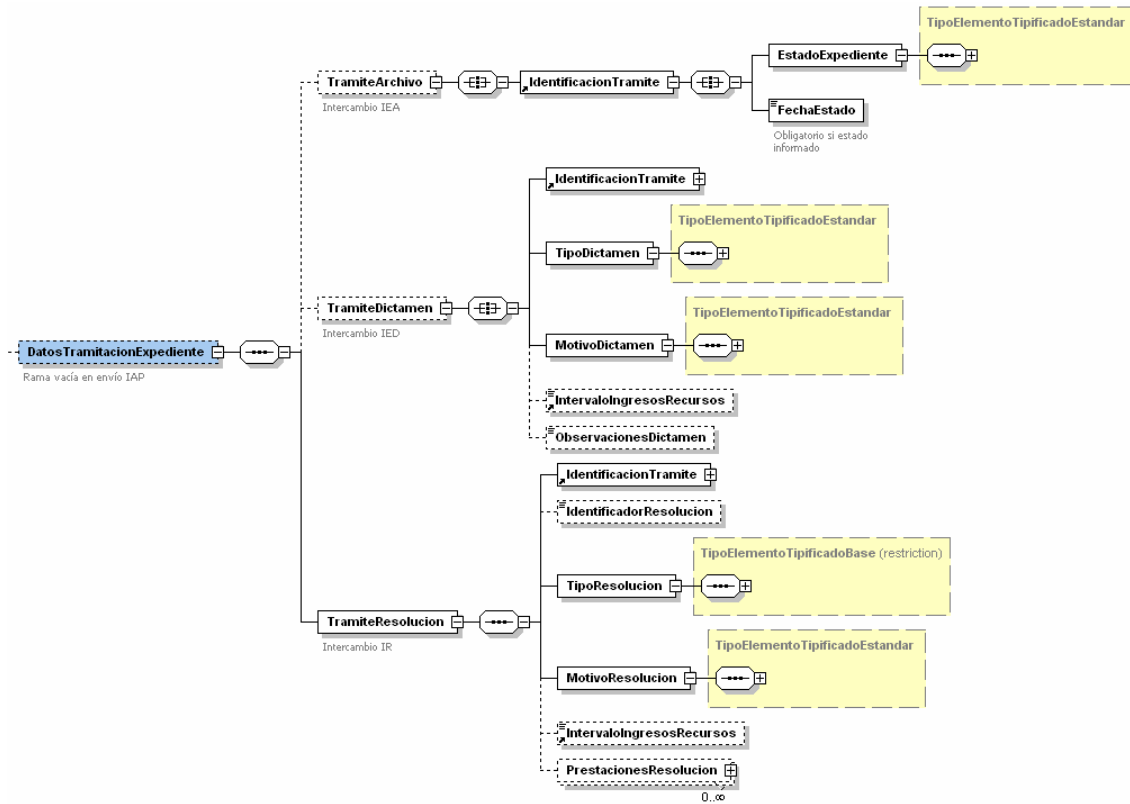
Figura 16. XSD-DatosTramitacionExpediente
