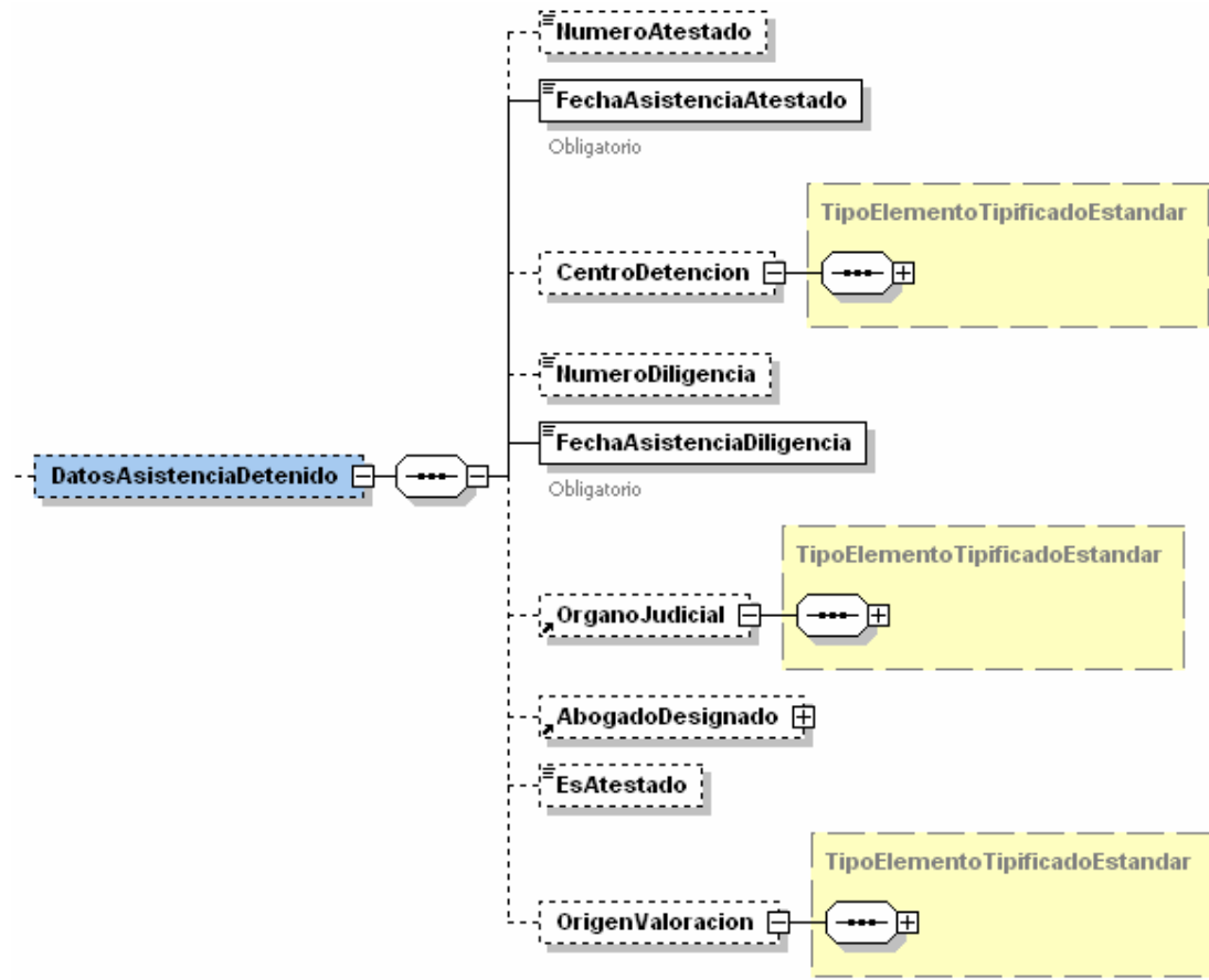
Figura 15. XSD-DatosAsistenciaDetenido
